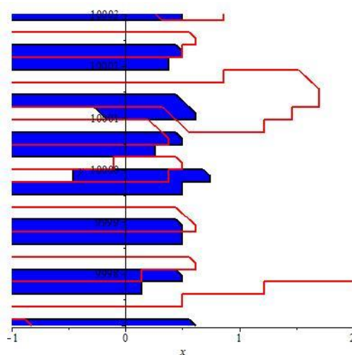
Рисунок 7 – График \text{Re}(\zeta(z)) < 0 , y_k \approx 10^4
