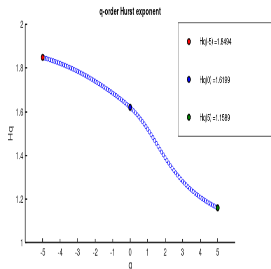
Рисунок 5 – Экспонента Херста для \text{density}=0,7
