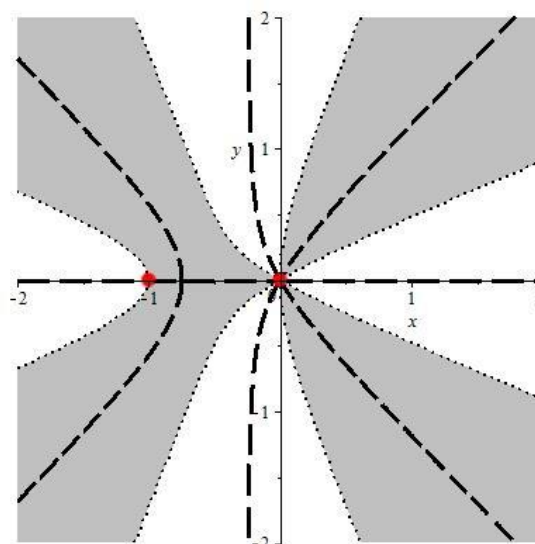
Рисунок 14 – 3-х кратный корень z^4 + z^3
