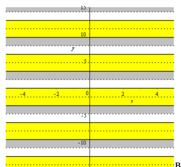
Рисунок 8 – Графики: а) \text{Re}(\exp(z)) < 0 ; б) \text{Im}(\exp(z)) < 0 ; в) на одном рисунке
