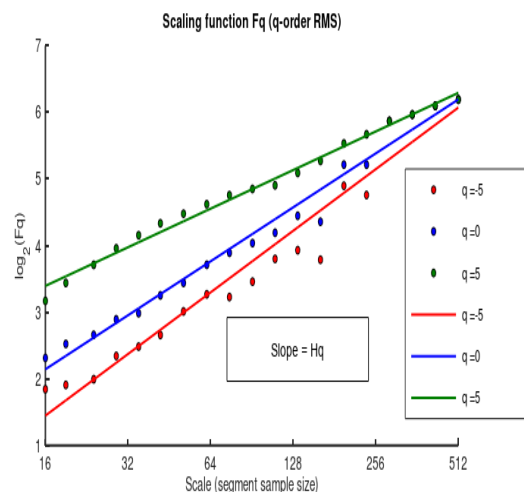
Рисунок 4 – Функция скейлинга для \text{density}=0,7
