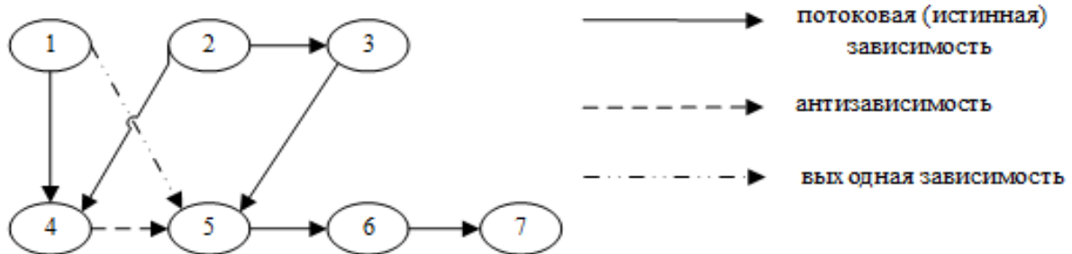
Рисунок 2 – Представление алгоритма в виде структурного графа
