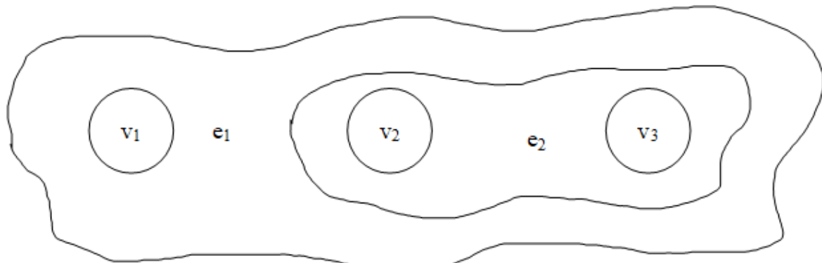
Рисунок 4 – Гиперграф
