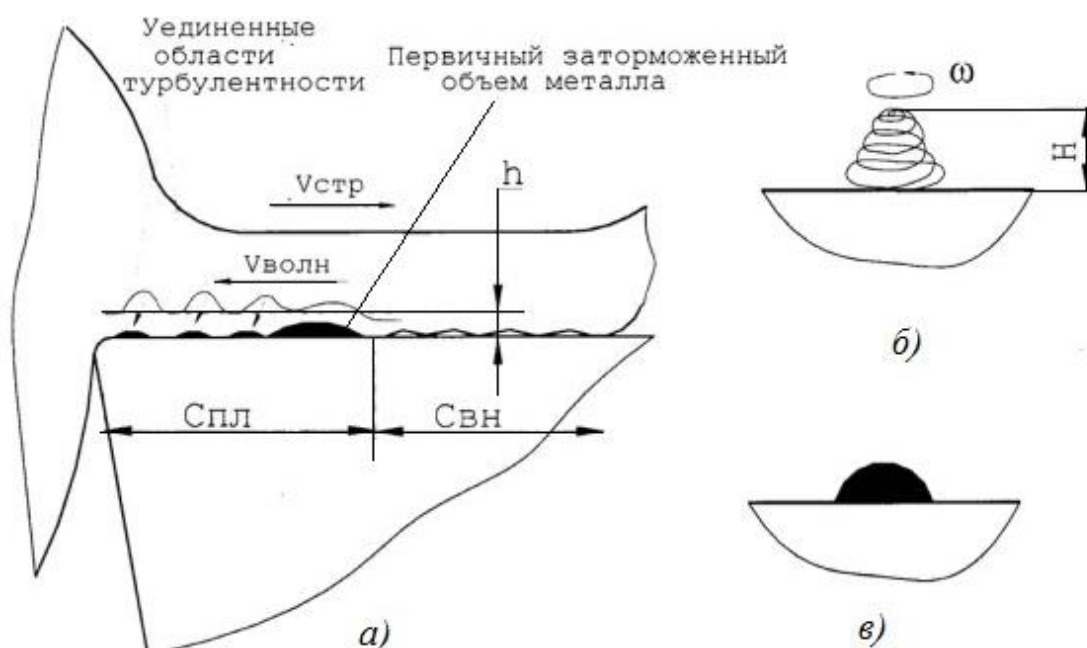
Рисунок 1. Схема образования нароста на передней поверхности инструмента: С_{пл} – длина зоны пластического контакта, С_{вн} – длина зоны внешнего контакта, h – толщина квазижидкого прирезцового слоя стружки, H – высота вихревого столба, \omega – угловая скорость вихря, V_{стр} – скорость стружки, V_{волн} – скорость волн.
